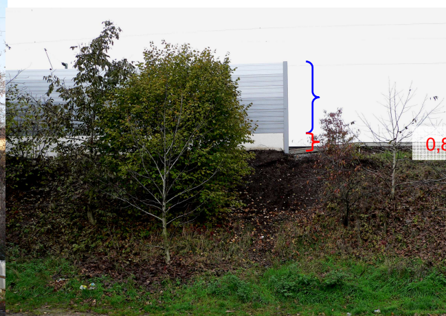
rechts: Im selben Maßstab angepasst LSW von Neuhermsheim (Foto: Nordabschluss)
